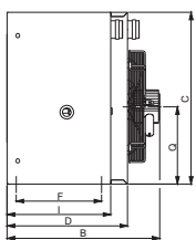
Right side view F2 60 - F2 80 - F2 100
