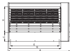
Front view F2 60 - F2 80 - F2 100
