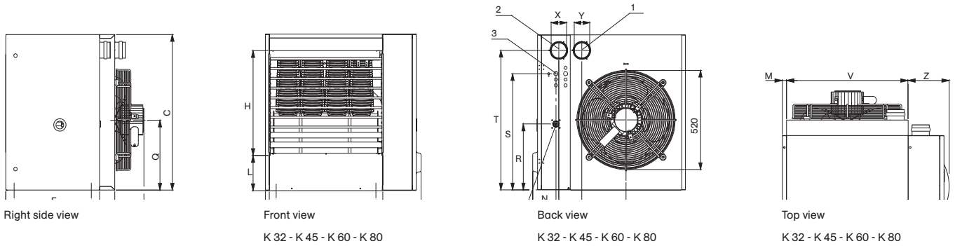
K 32 - K 45 - K 60 - K 80
