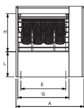
Front view F1 21 - F1 31 - F1 41 - F1 51
