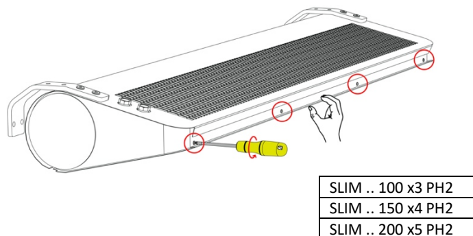
RYS. 11.2 ODKRĘCENIE ŚRUB OD FRONTU.
