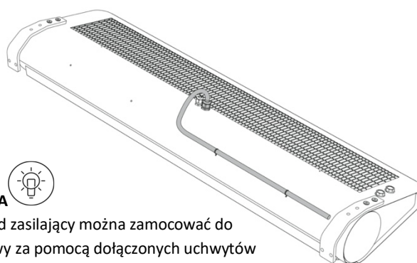
RYS. 11.6 PROWADZENIE PRZEWODU PO OBUDOWIE.
