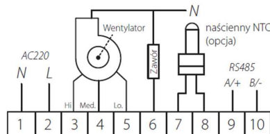
Schemat podłączeniowy NTC do sterownika HMI
