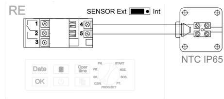
Schemat podłączeniowy NTC do termostatu RE
