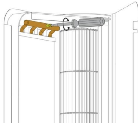
РИС. 17.2 ВСТРОЕННЫЙ КЛАПАН.
