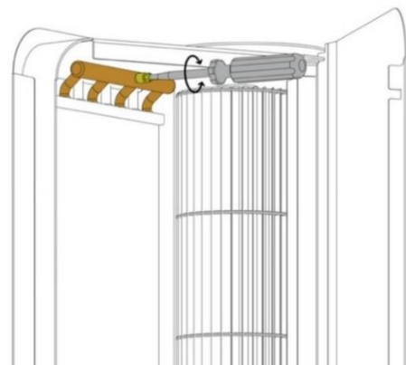
RYS. 17.2. WBUDOWANY ZAWÓR ODPOWIERZAJĄCY.
