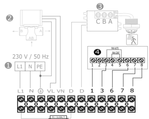
СХЕМА 15.2. SLIM-W/N + TS
