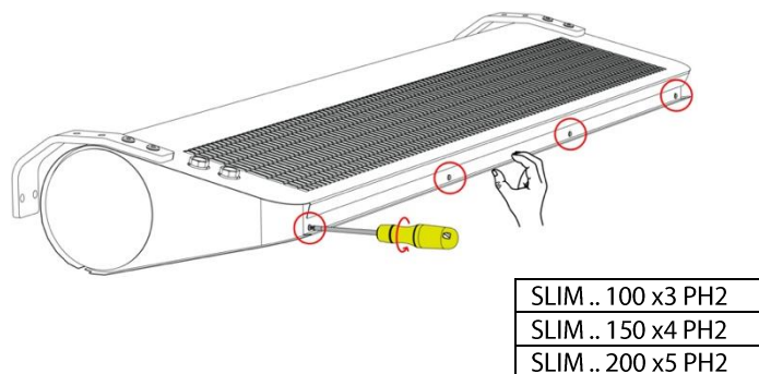
RYS. 11.2 ODKRĘCENIE ŚRUB OD FRONTU.
